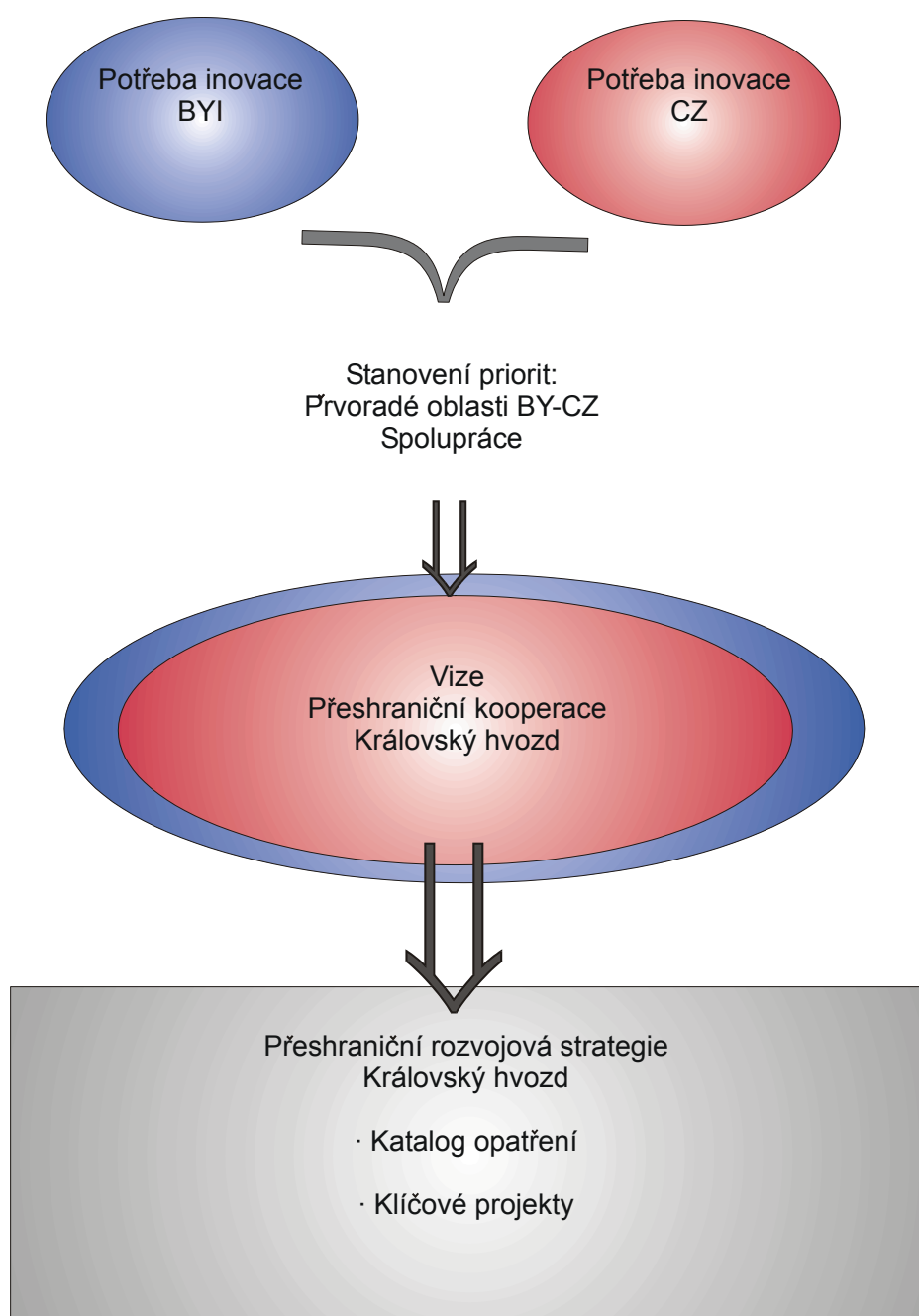
Obr. 3 Metodický postup
